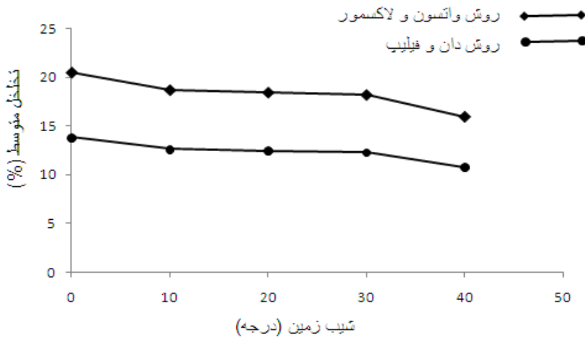
شکل ۳- تغییرات مقدار تخلخل متوسط با تغییرات شیب زمین
