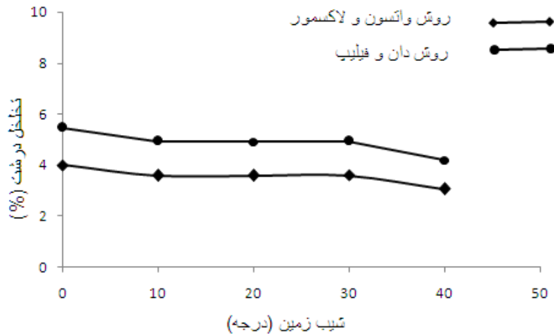
شکل ۲- تغییرات مقدار تخلخل درشت با تغییرات شیب زمین
