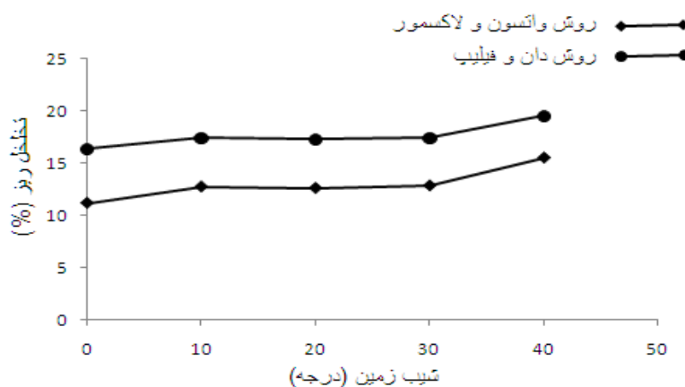
شکل ۴- تغییرات مقدار تخلخل ریز با تغییرات شیب زمین
