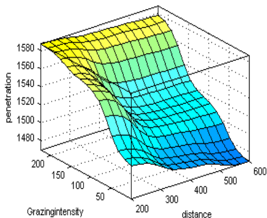
شکل ۸: پیش‌بینی نفوذپذیری خاک (کیلو پاسکال) در ارتباط با فاصله از روستا (متر) و شدت‌های چرایي توسط انفیس
