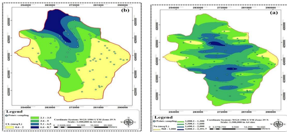
Fig. 5 - Zoning (a) Na changes and zoning (b) Cl changes Ardabil plain شکل ۵- پهنه‌بندی (a) تغییرات Na و پهنه‌بندی (b) تغییرات Cl دشت اردبیل
