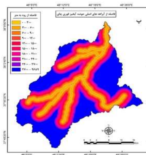
شکل ۳: توزیع فضایی پارامترهای هیدرولوژیکی در سطح حوضه قوری چای (منبع: نویسندگان، ۱۳۹۸)
