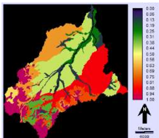
شکل ۱۴: نقشه فازی لایه سازندهای زمین‌شناسی
