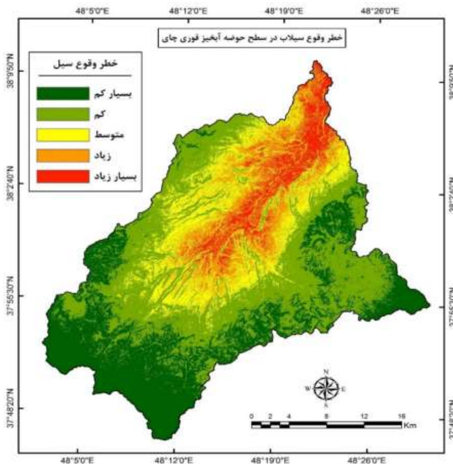
شکل ۱۵: پهنه‌بندی خطر سیلاب در سطح حوضه آبخیز قوری چای با استفاده از مدل ANP
