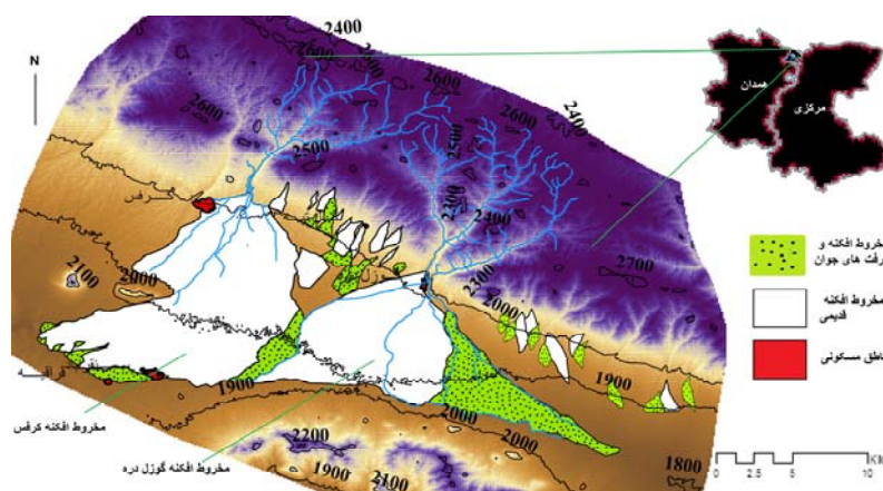
شکل ۱: موقعیت مخروط‌افکنه‌های منطقه
