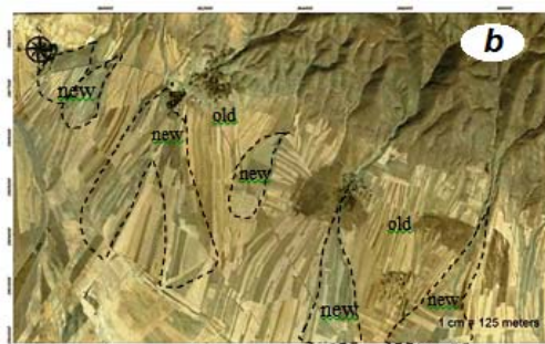
شکل ۲: ا- (موقعیت ۱ در شکل ۱) انتقال محل شکل گیری مخروطافکنه جدید (با رنگ روشن و با حرف (new) در قسمت پایینی نشان از آرامش تکتونیکی جبهه کوهستان دارد. در این صورت شبکه آبراهه تمایل دارد رسوبات را در قسمت پایینی مخروطافکنه قدیمی (old) نهشته کند. ب- (موقعیت شماره ۲) با حرکت به طرف شرق محدوده مخروطافکنه های جدید در حال پیشروی به طرف جبهه کوهستان هستند. که نشانه ی بالا آمدن جبهه کوهستان در اثر فعالیت تکتونیکی است. ۱
