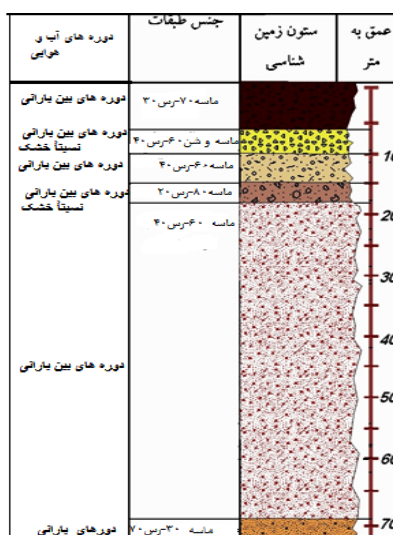
شکل ۴: لوگ زمین‌شناسی از مخروط‌افکنه کرفس در حاشیه‌ی روستای سنقرآباد. رسوبات ریزدانه معرف دوره‌های بارانی و سرد که در قسمت پایین لوگ قرار دارد و رسوبات با دانه‌های درشت در قسمت‌های بالایی لوگ که معرف دوره‌ی بین یخچالی و گرم هولوسن قرار دارد. مأخذ: وزارت نیرو، ۱۳۹۰
