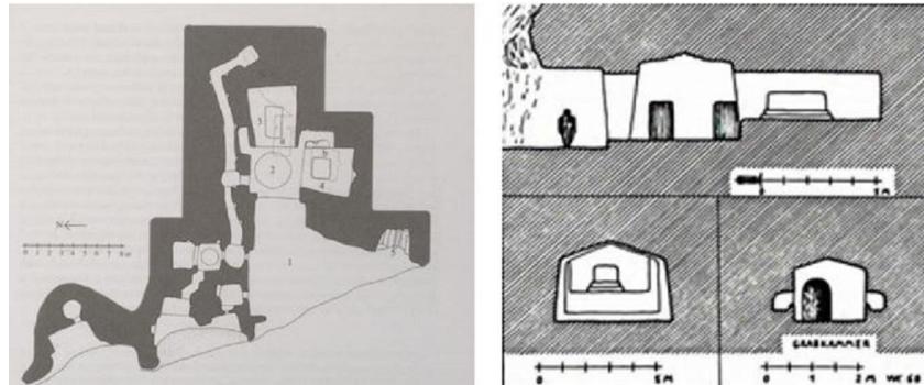
شکل ۲. (راست) مقطع قسمت اصلی نیایشگاه مجموعه صخره‌ای رصدخانه (Kleiss, 1969: 51)؛ (چپ) پلان مجموعه صخره‌کند تپه رصدخانه (Ball, 1976).
