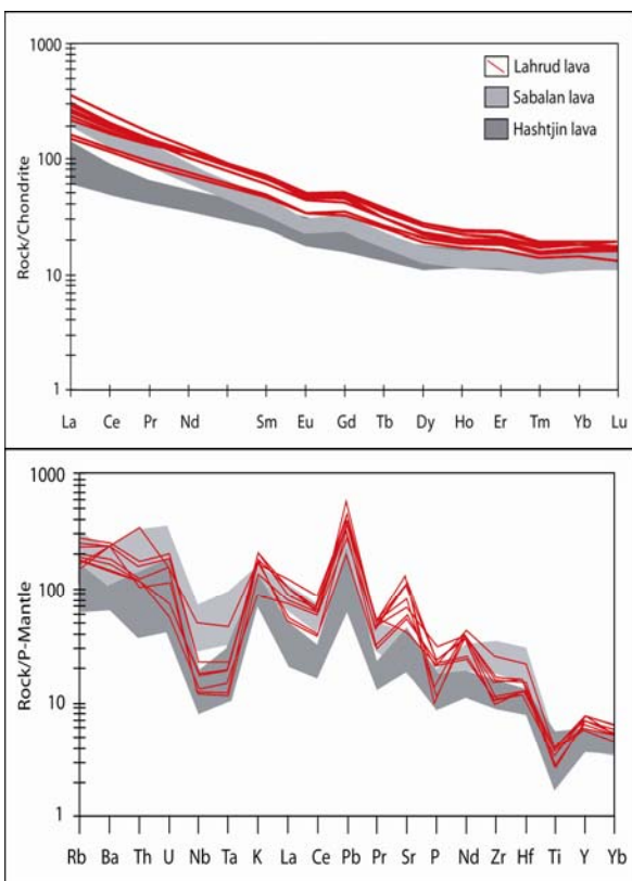
شکل ۷- دیاگرام عناصر نادر خاکی نرمالیز شده نسبت به کندریت و دیاگرام عناصر کمیاب نرمالیز شده نسبت به گوشته اولیه برای سری‌های ولکانیکی منطقه لاهرود، سبلان و هشتجین
