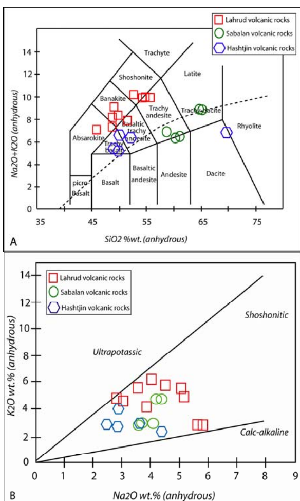
شکل ۵- ترکیب ولکانیک‌های مورد مطالعه (محدوده‌های لاهرود، سبلان و هشتجین) در: (A) دیاگرام مجموع آلکالی‌ها در مقابل اکسید سیلیس (LeBas et al. , 1986) (B) دیاگرام اکسید پتاسیم در مقابل اکسید سدیم (Chung et al. , 1998) (مقادیر اکسید سیلیسیم، اکسید پتاسیم و اکسید سدیم بر حسب مقادیر خشک و بی‌آب محاسبه شده است)
