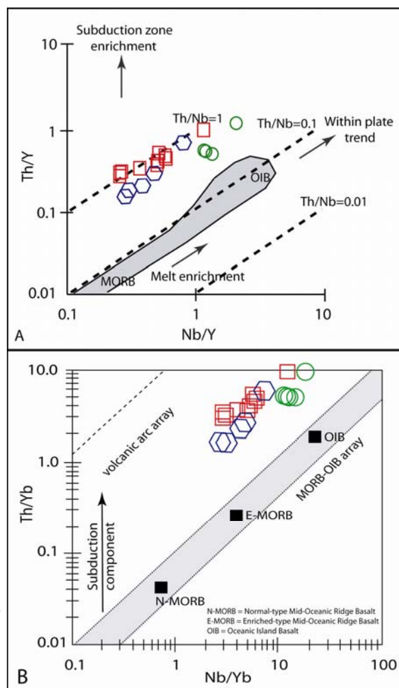
شکل ۸- ولکانیک‌های مورد مطالعه بر روی: (A) دی‌گرام Th/Y مقابل Nb/Y (B) دی‌گرام Th/Yb مقابل Nb/Yb (Alichi et al., 2002). (با اندکی تغییرات). (Leat et al., 2004)
