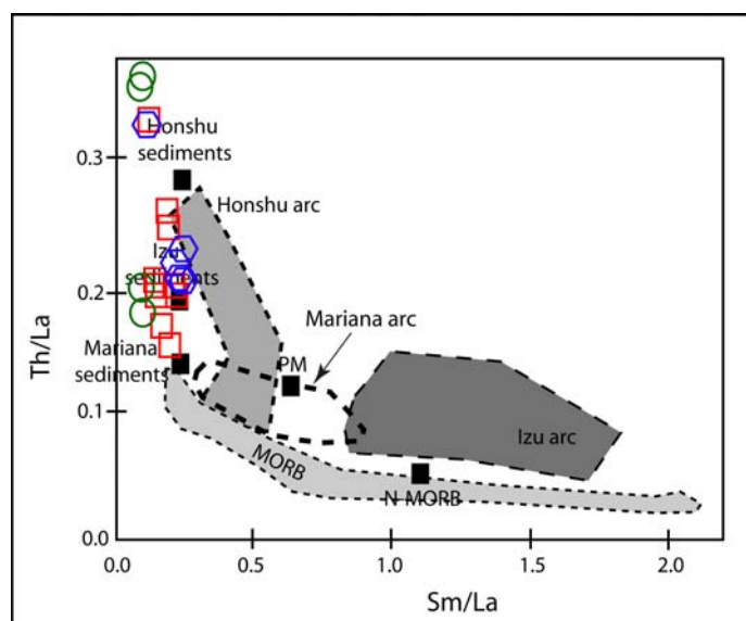
شکل ۹- دیاگرام Th/La در مقابل Sm/La برای بازالت‌های قوس‌های آتشفشانی و سری‌های ولکانیکی منطقه مورد مطالعه (با تغییرات از Plank و همکاران، ۲۰۰۷). هر قوس آتشفشانی روندی اختلاطی (Mixing trend) بین یک ترکیب گوشته‌ای (در آرایش MORB در حوضه خاکستری رنگ) و یک ترکیب رسوبی (رسوبات دراز گودال) را تشکیل می‌دهد.
