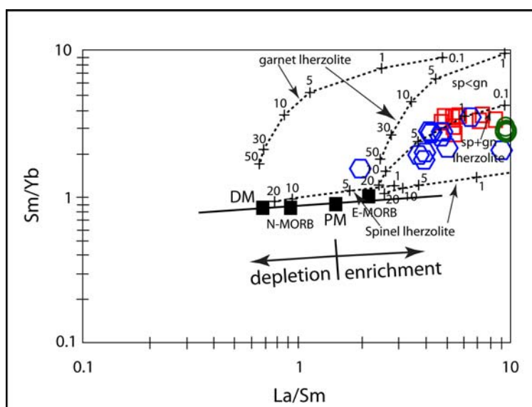
شکل ۱۰- تغییرات عناصر نادر خاکی در سری‌های ولکانیکی مورد مطالعه بر حسب دیاگرام Sm/Yb در مقابل La/Sm. روند گوشته‌ای (Mantle array) در این شکل (خط ضخیم) توسط ترکیب گوشته تهی شده تیپ مورب (DM) (McKenzie and O'Nions, 1991) و گوشته اولیه (PM) (Sun and McDonough, 1989) مشخص می‌شود. منحنی‌های ذوب‌بخشی برای منشأ گوشته‌ای اسپینل لروزولیت ( Ol_{53}+Opx_{27}+Cpx_{17}+Sp_{11} ) و گارنت لروزولیت ( Ol_{60}+Opx_{20}+Cpx_{10}+gt_{10} ) با ترکیبات گوشته تهی شده تیپ مورب و گوشته اولیه از Aldanmaz و همکاران (۲۰۰۰)، افزون بر این، خطوط و اعداد روی منحنی‌های ذوب نشان‌دهنده درجه ذوب‌بخشی برای یک منشأ گوشته‌ای باشد. علاوه بر این، در این دیاگرام ترکیب N-MORB و E-MORB از Sun و McDonough (۱۹۸۹) نیز آورده شده است.
