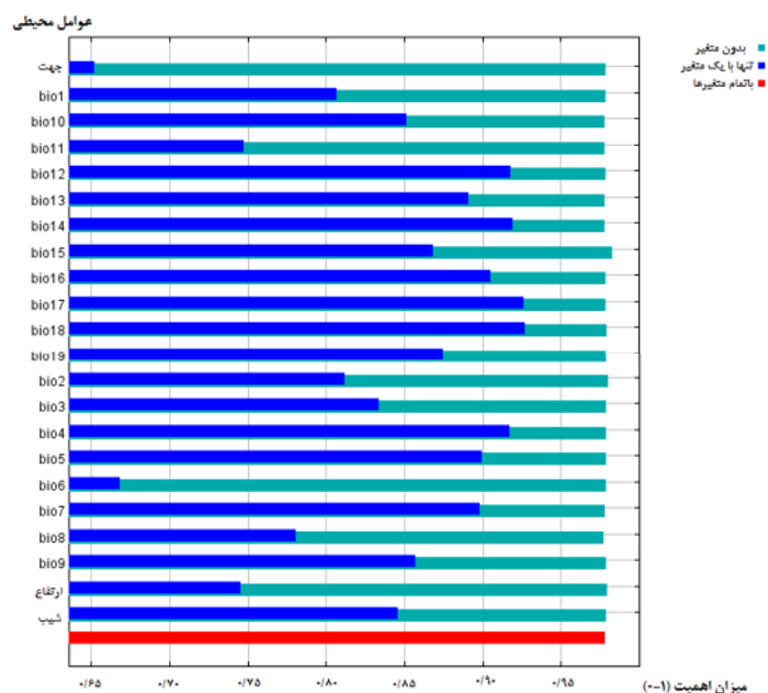
شکل ۵: نتایج حاصل از روش چک‌نایف در ارتباط با اهمیت متغیرهای محیطی در منطقه مورد مطالعه
