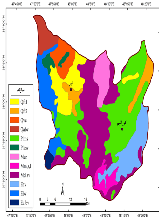
زمین‌شناسی
