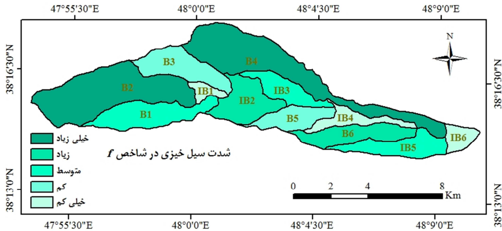
شکل ۹: شدت سیل خیزی زیرحوزه‌های حوزه آبخیز عموقین بر اساس رتبه‌بندی شاخص f
