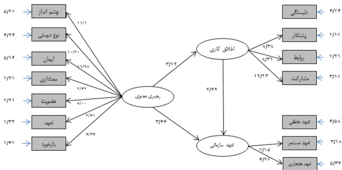
نگاره ۲. اعداد معنی داری مدل ساختاری پژوهش
