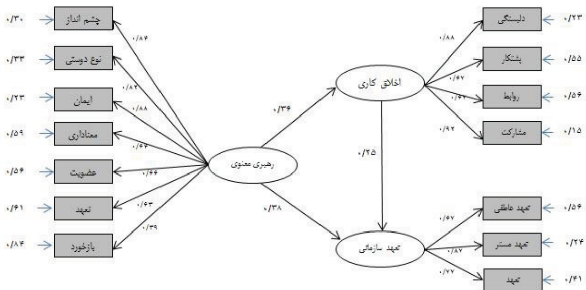
نگاره ۱. ضرایب تخمین استاندارد مدل ساختاری پژوهش
