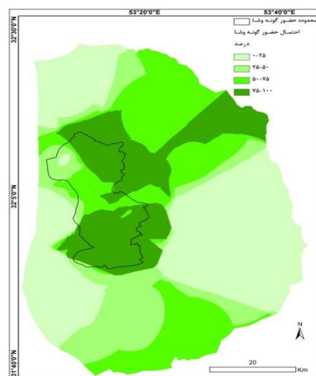
شکل ۳- احتمال حضور گونه D. ammoniacum D. DON. در رویشگاه ندوشن
