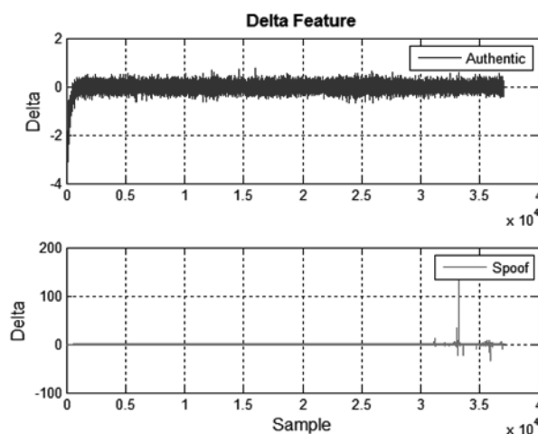
شکل (۵). ورودی اول شبکه عصبی پیشنهادی (شاخص دلتا).
