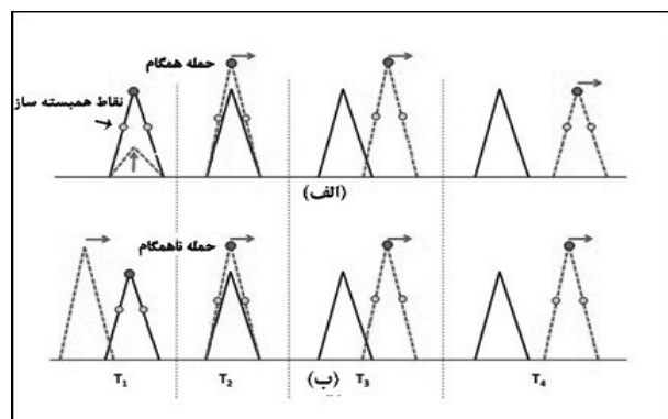
شکل (۲). دو سناریوی فریب، شکل ناحیه همبستگی در حلقه ره‌گیری: (الف) فریب همگام و (ب) فریب ساده [۸].
